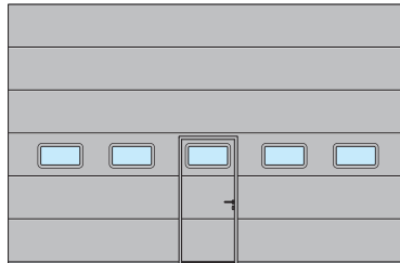
SPU F42 Lamelli-ikkunat, tyyppi E Käyntioven sijoittelu keskelle
