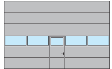
SPU F42, SPU 67 Thermo Alumiiniset ikkunakehykset Käyntioven sijoittelu keskelle
