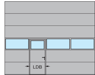
SPU F42, SPU 67 Thermo Alumiiniset ikkunakehykset Käyntioven sijoittelu vasemmalle
