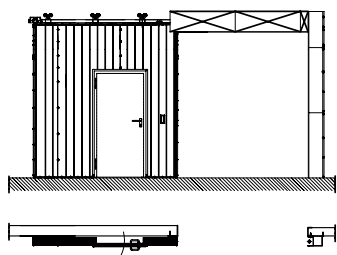
Paloliukuovi 2-puoleinen, kun aukon kummallakkaan sivuilla ei ole riittävästi levyttä yksilehtiselle ovelle
