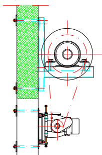
Moottorin kiinnitys
