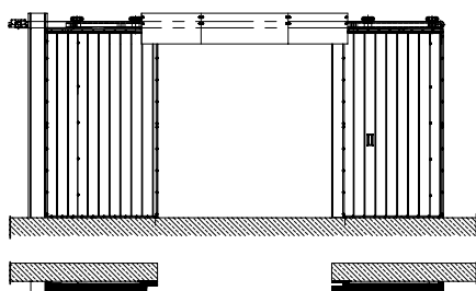
Paloliukuovi 2-puoleinen, kun aukon kummallakkaan sivuilla ei ole riittävästi levyttä yksilehtiselle ovelle
