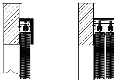
Suojattu liukujärjestelmä palotilanteessa
