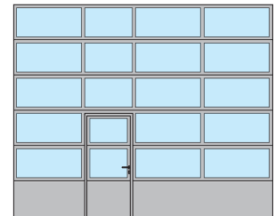
APU F42, APU F42 Thermo, APU 67 Thermo Käyntioven sijoittelu vasemmalle
