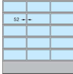
APU F42, APU F42 Thermo, APU 67 Thermo Tasainen kenttäjako
