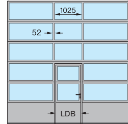
APU F42, APU F42 Thermo, APU 67 Thermo Käyntioven sijoittelu keskelle
